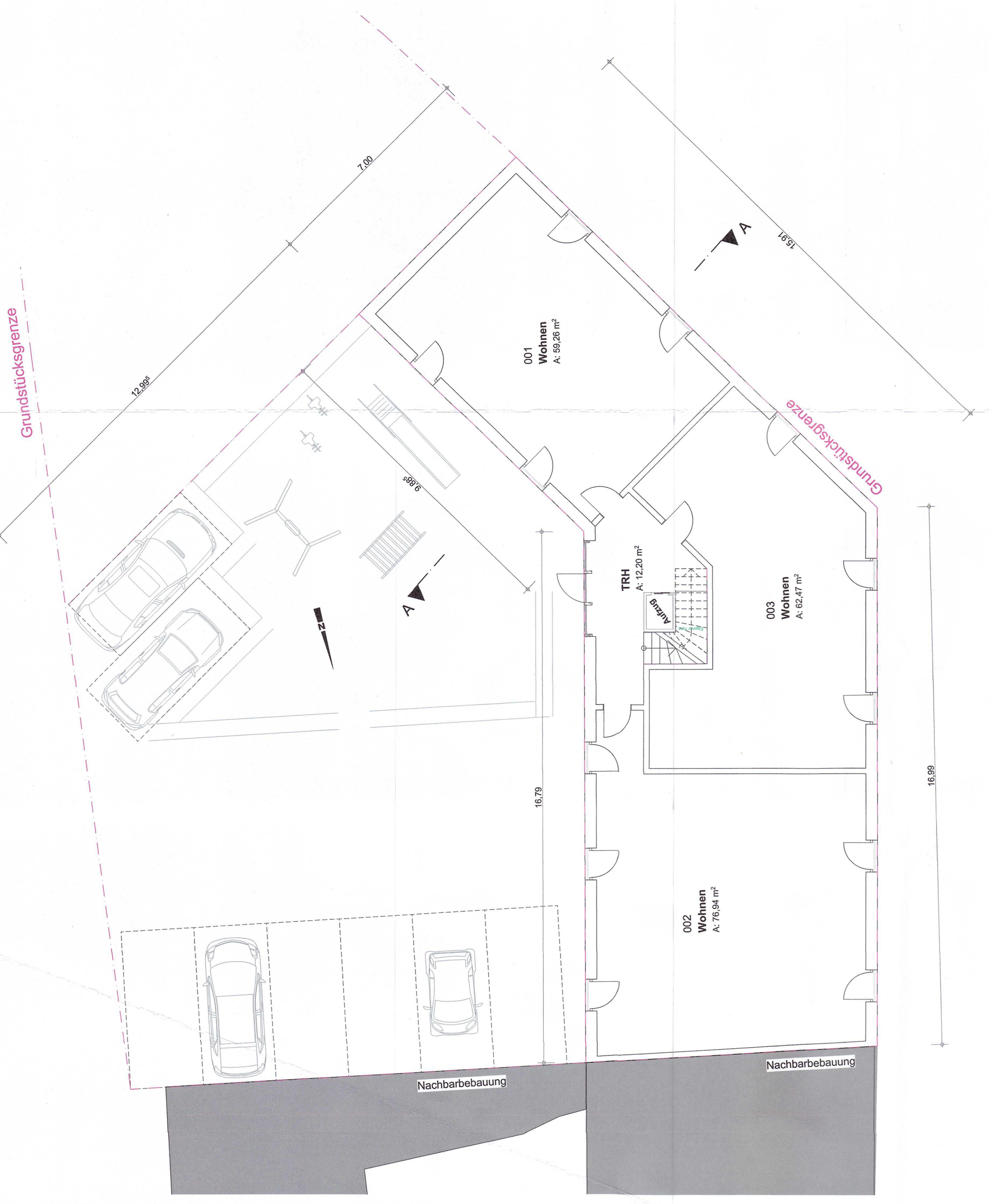
Grundriss EG, M 1:100
