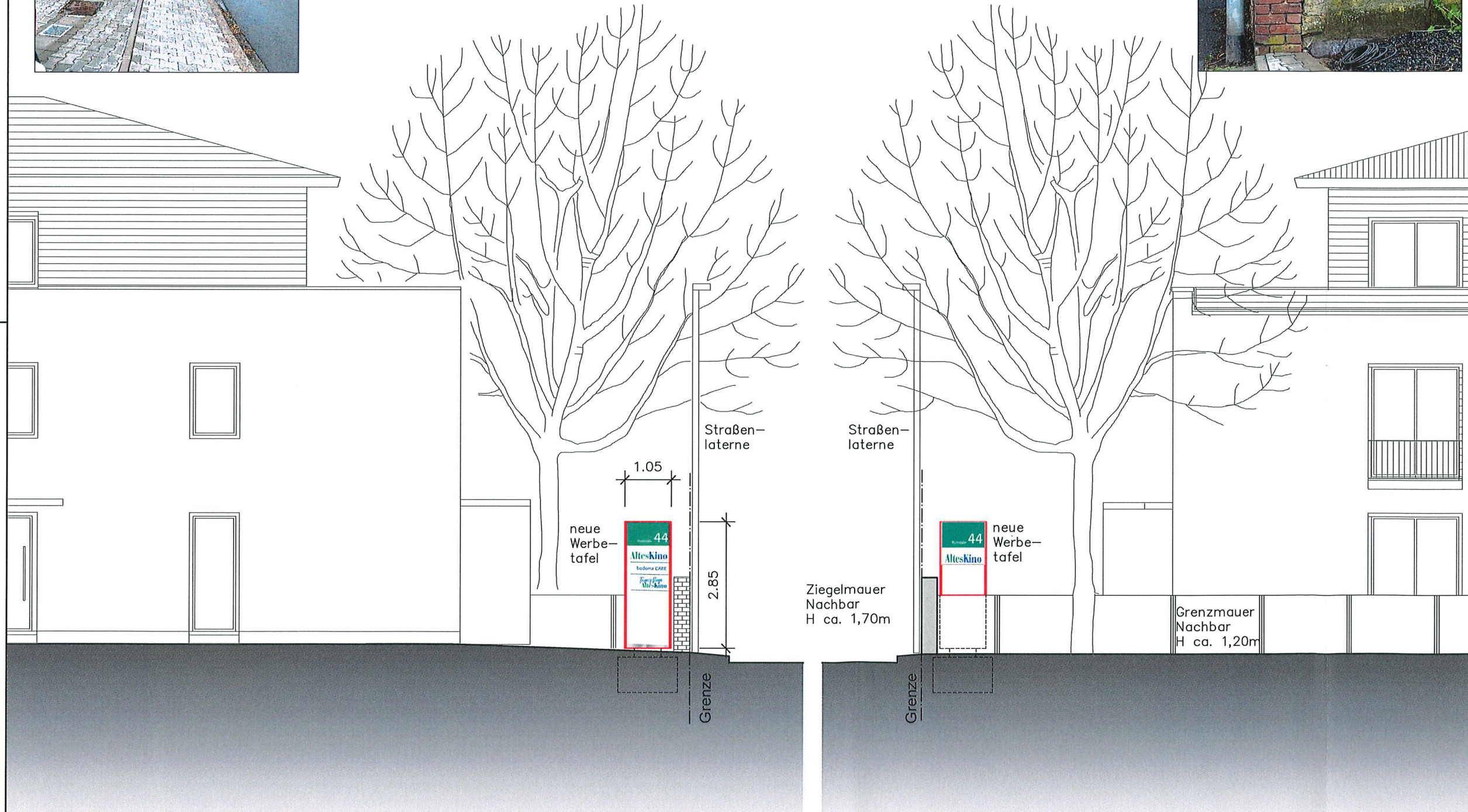
Nordansicht Südansicht
