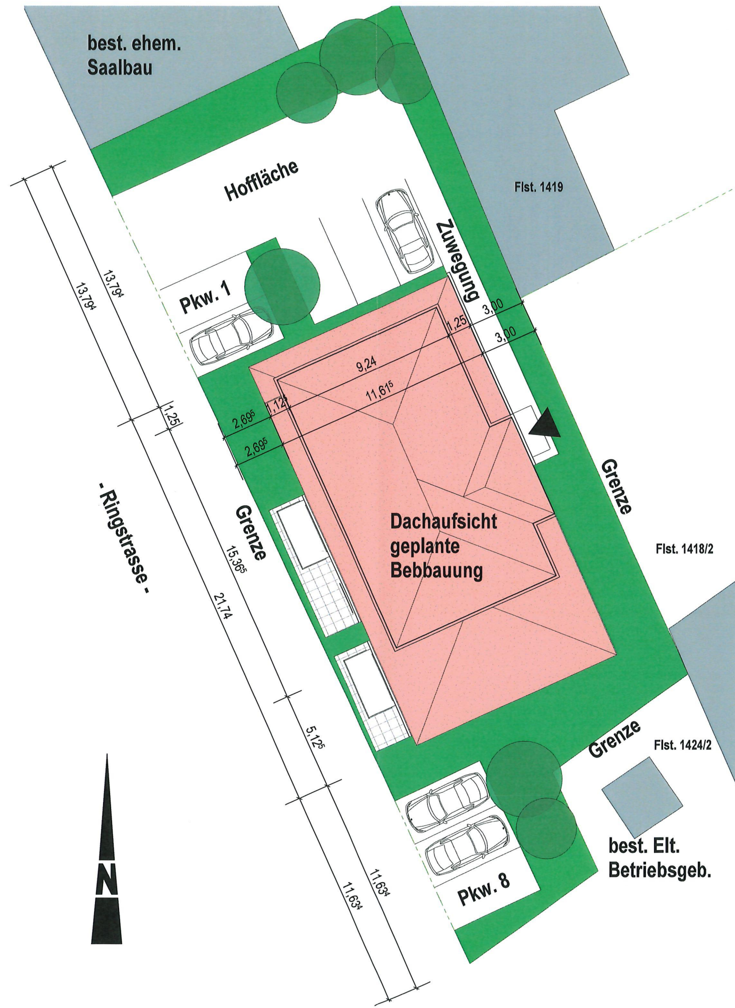
Flächengestaltungsplan M 1 : 200
