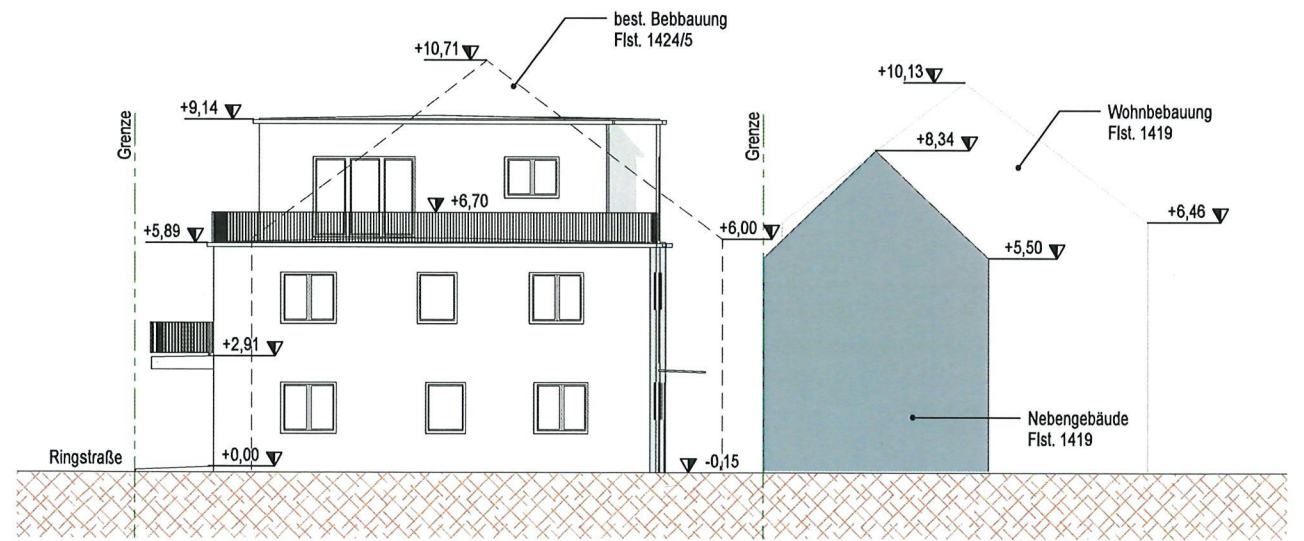
Südansicht M 1 : 200
