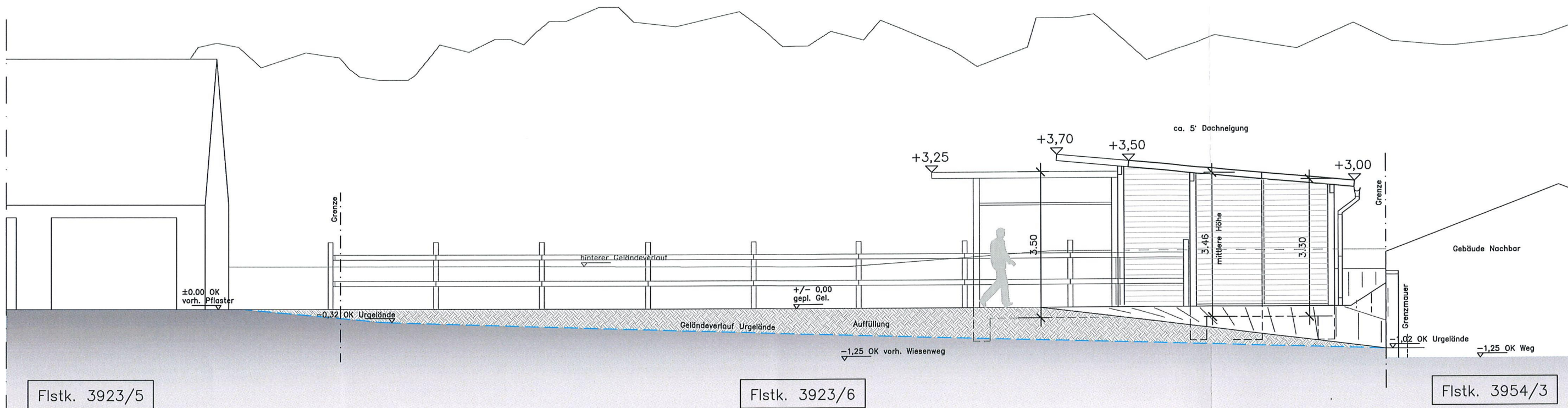
SÜD-OST-ANSICHT
