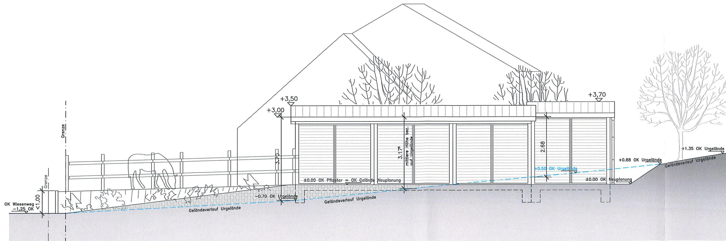
NORD-OST-ANSICHT
