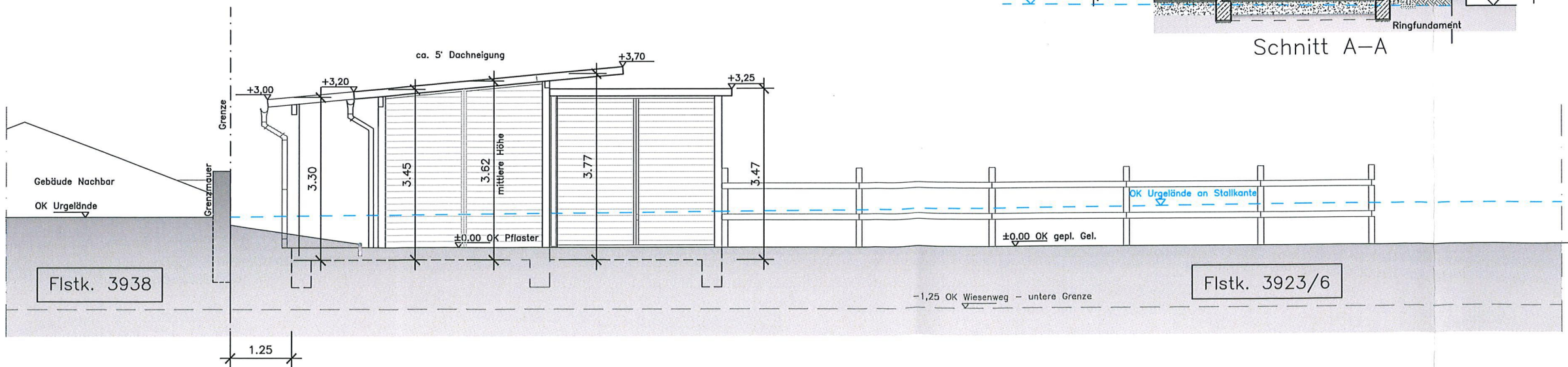
NORD-WEST-ANSICHT
